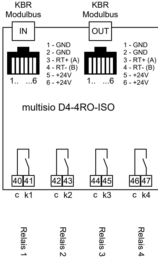
Abb. 1: Anschlussplan D4-4RO-ISO
